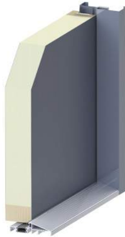
75 PASSIVE (zewnątrzne)
