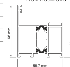
Profil naświetla
