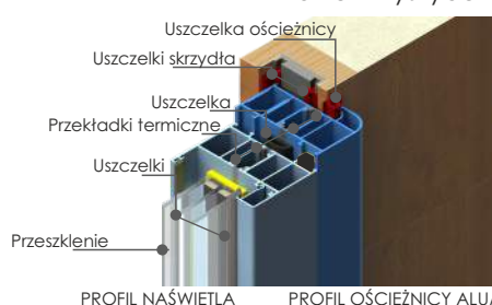
Pakiet trzyszybowy
