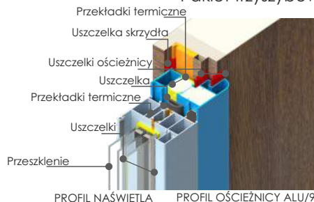
Pakiet trzyszybowy
