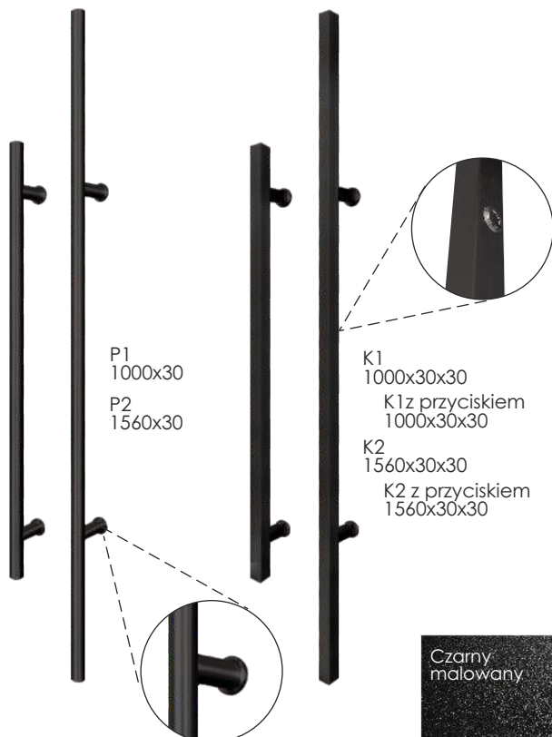
POCHWYT OKRĄGŁY
