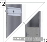
Elementy wzmacniające konstrukcję ościeznicy z kotwami montażowymi lub bez 12. Ościeznica 10/54,11/54 13. Ościeznica 15/54
