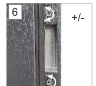
Dwie regulacje docisku rygli +/-
