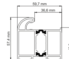
Profil ościeżnicy ALU/54
