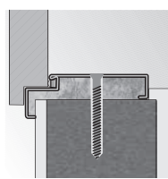
ościeznica Kątowa DUŻA montaż na dyble
